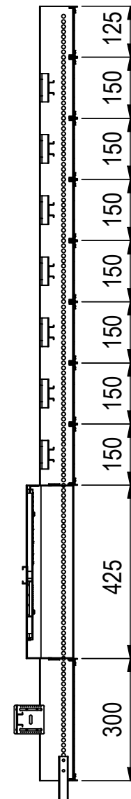
A-A ( 1 : 13 )
