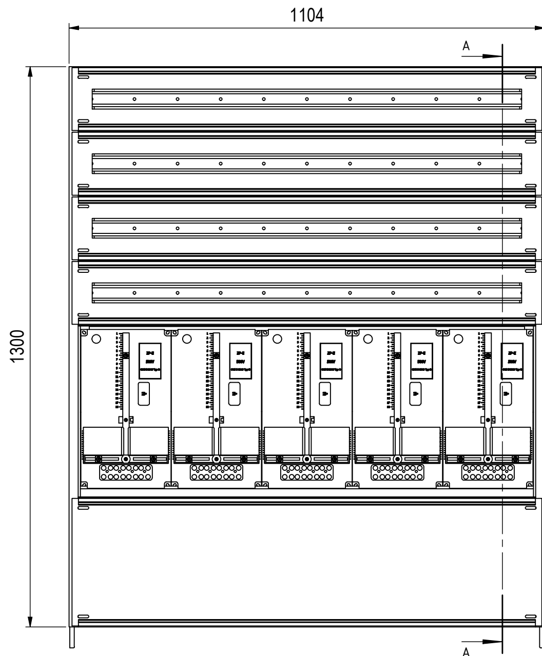
Hutschiene Vorzählerfach 1049
