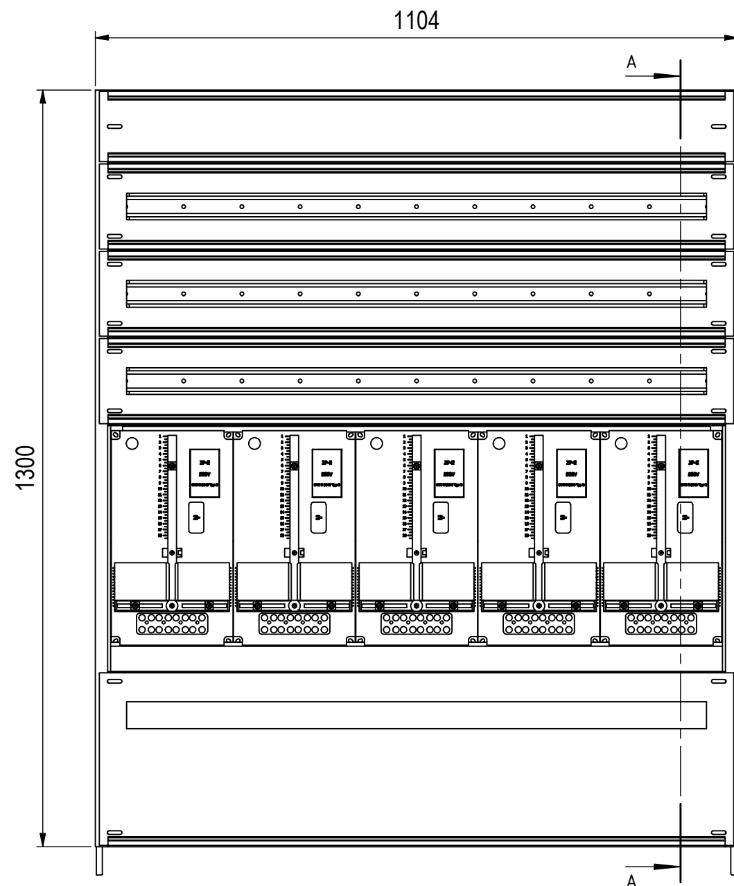
Hutschiene Vorzählerfach 1049
