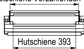
Hutschiene Vorzählerfach 429
