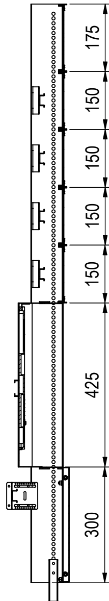
A-A ( 1 : 10 )
