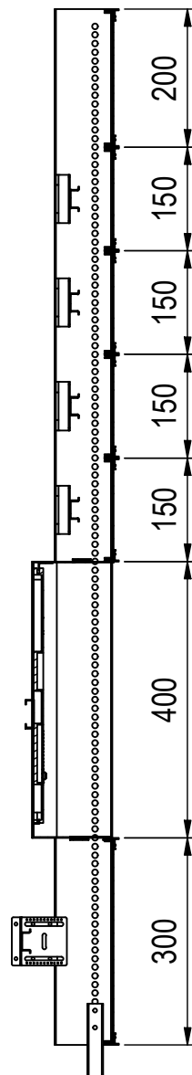
A-A ( 1 : 10 )
