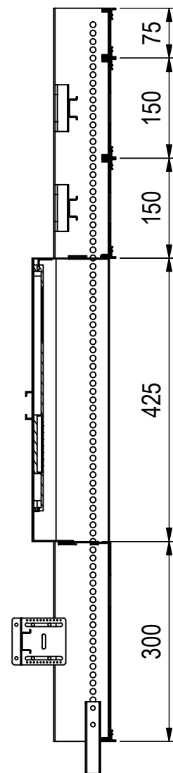
A-A ( 1 : 8 )
