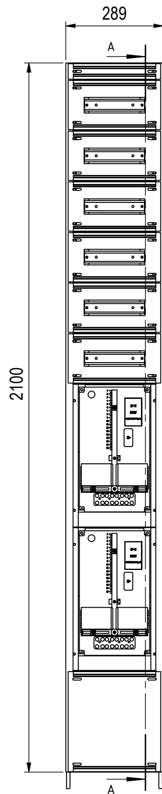
Hutschiene Vorzählerfach 214
