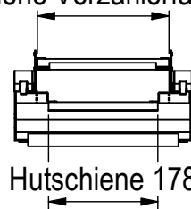
Hutschiene Vorzählerfach 214
