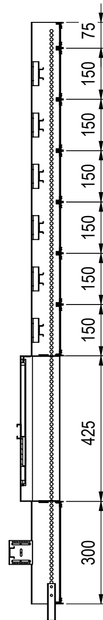
A-A ( 1 : 11 )
