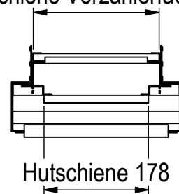
Hutschiene Vorzählerfach 214
