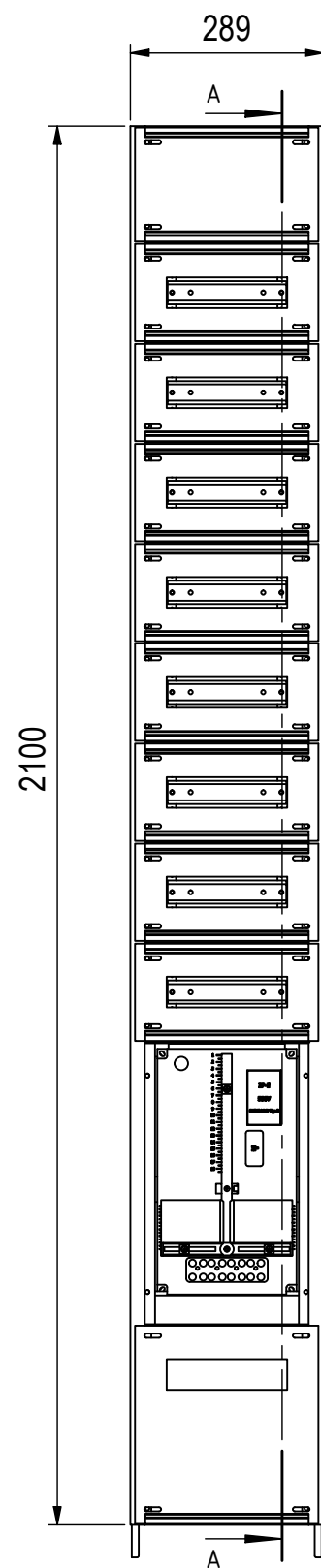
Hutschiene Vorzählerfach 214
