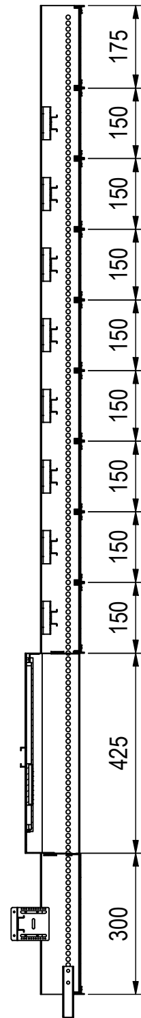
A-A ( 1 : 11 )
