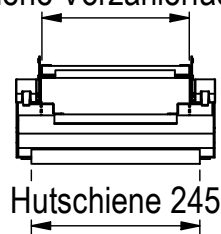
Hutschiene Vorzählerfach 214
