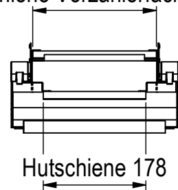
Hutschiene Vorzählerfach 214
