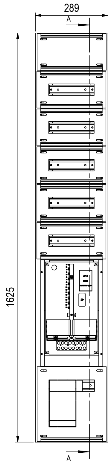
Hutschiene Vorzählerfach 214
