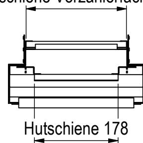
Hutschiene Vorzählerfach 214
