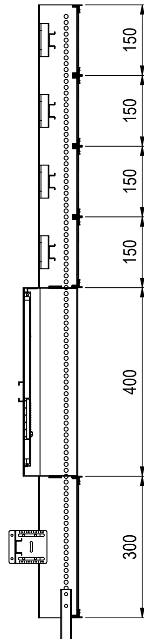
A-A ( 1 : 8 )
