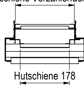
Hutschiene Vorzählerfach 214
