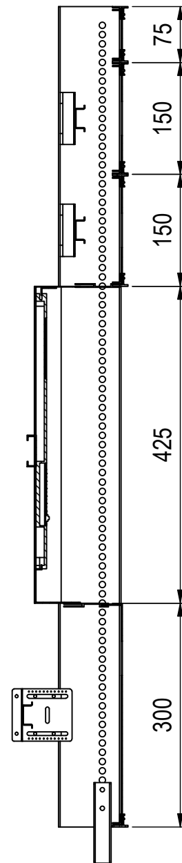
A-A ( 1 : 7 )
