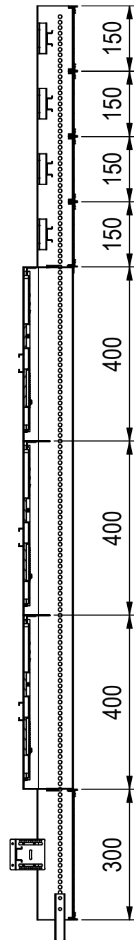
A-A ( 1 : 12 )
