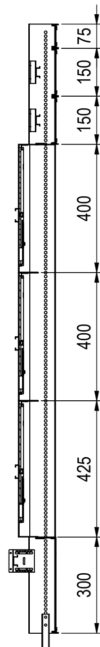
A-A ( 1 : 12 )
