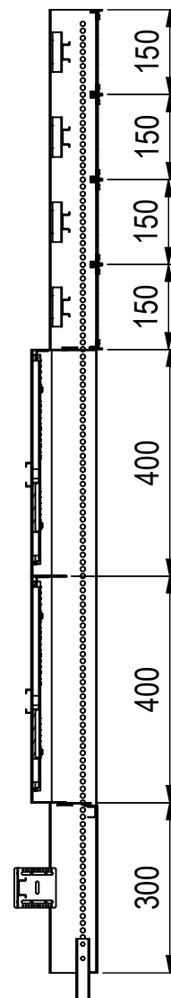
A-A ( 1 : 12 )
