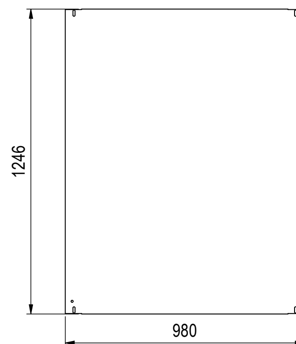
Montageplatte ( 1 : 15 )
