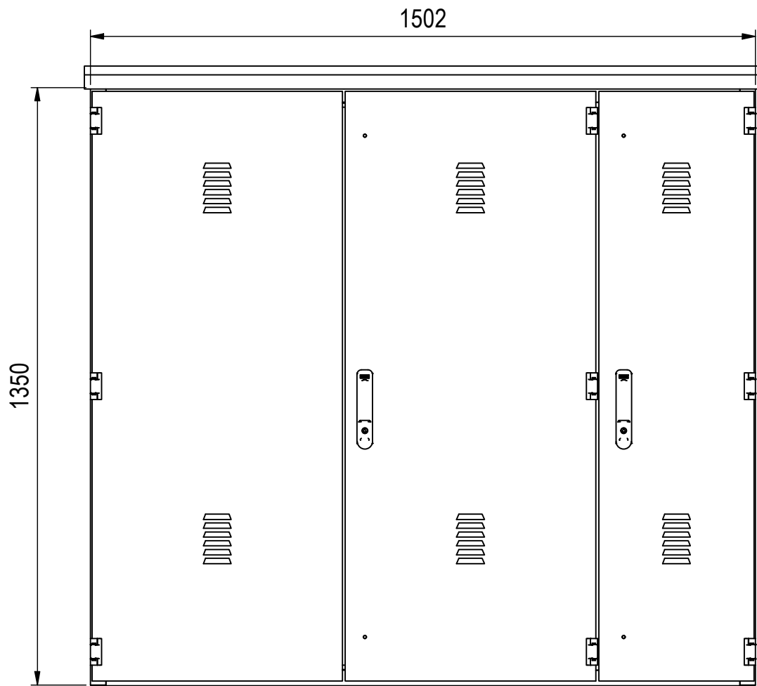
Innenschrank ( 1 : 12 )
