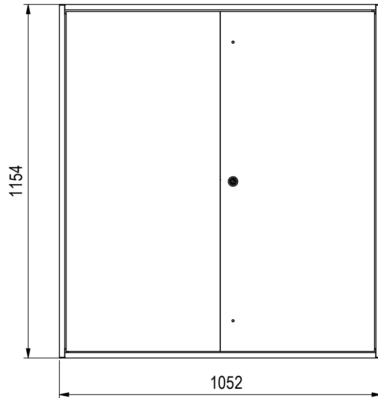
Innenschrank ( 1 : 12 )
