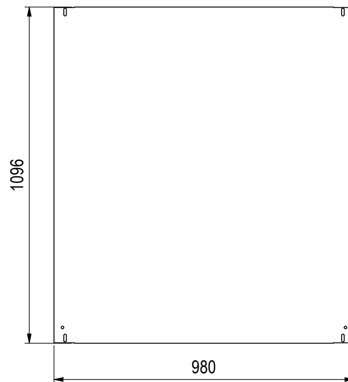
Montageplatte ( 1 : 12 )
