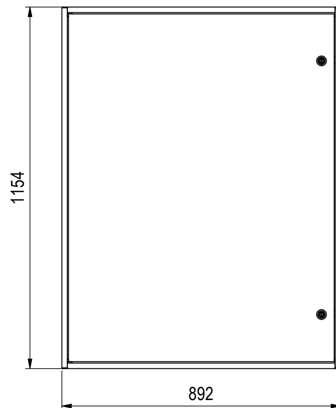
Innenschrank ( 1 : 12 )
