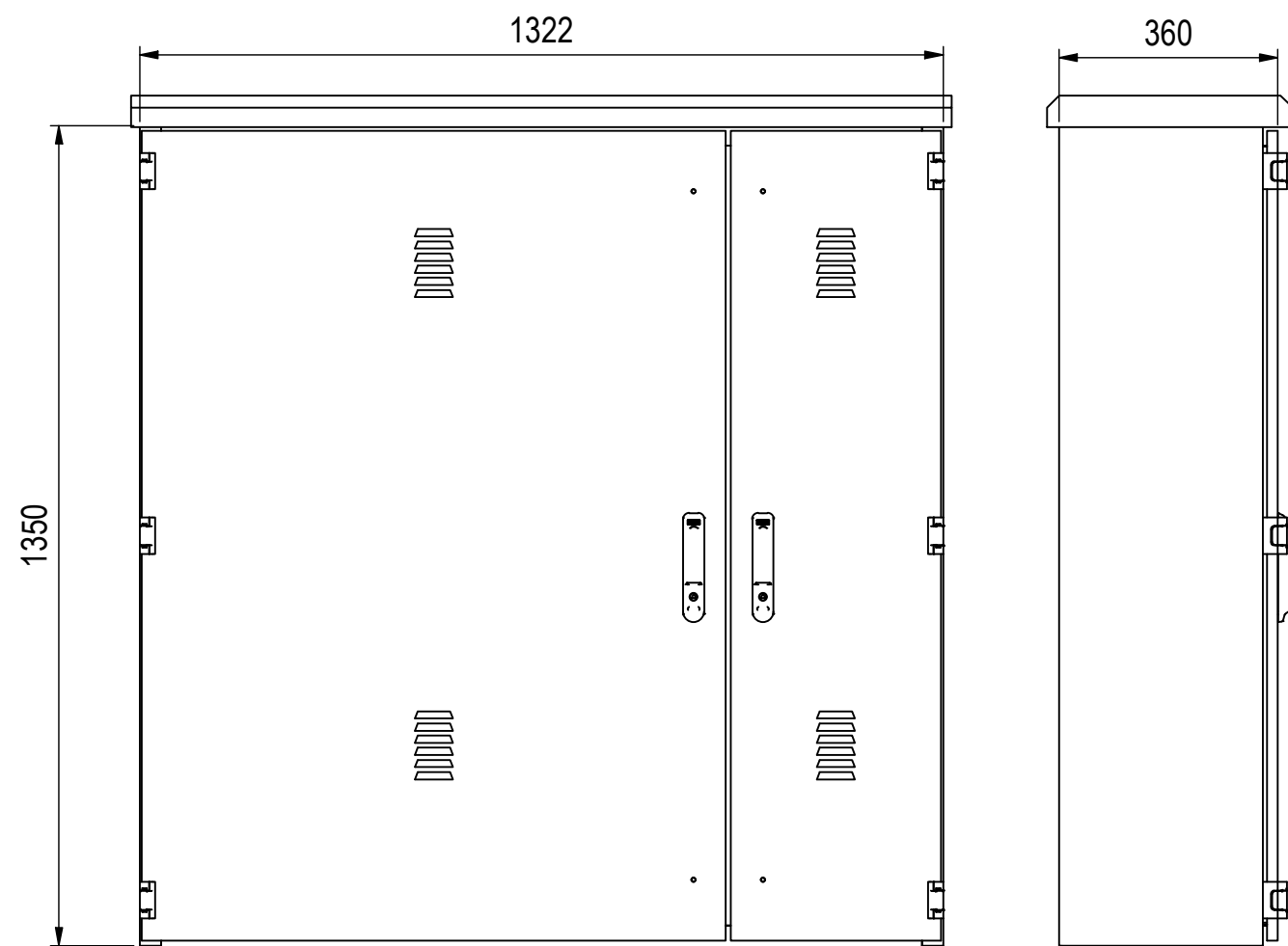
Innenschrank ( 1 : 12 )
