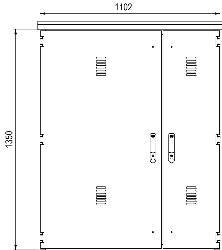
Innenschrank ( 1 : 12 )
