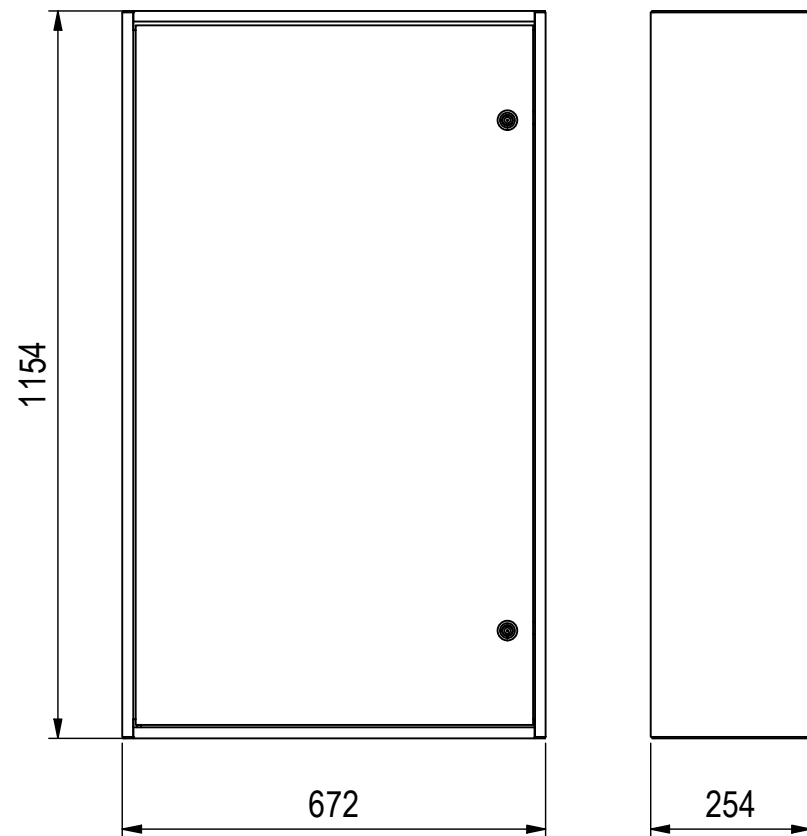
Innenschrank ( 1 : 12 )
