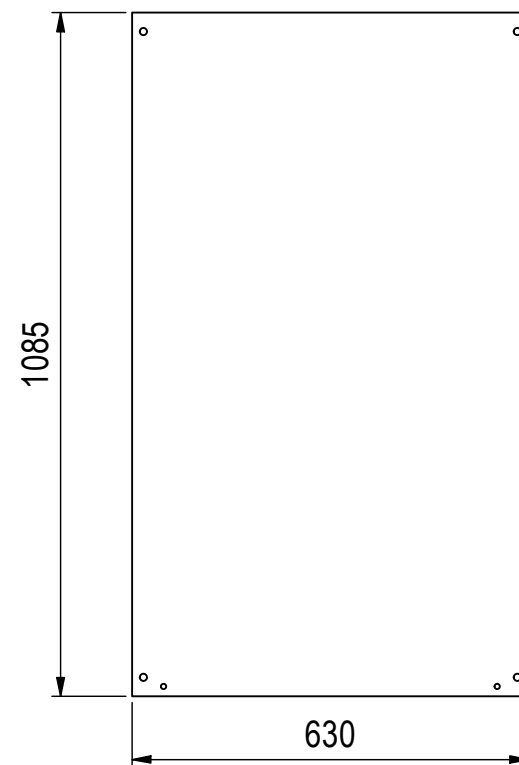
Montageplatte ( 1 : 12 )
