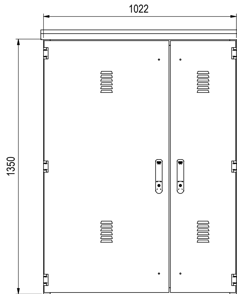
Innenschrank ( 1 : 12 )
