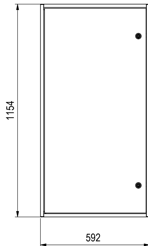
Innenschrank ( 1 : 12 )
