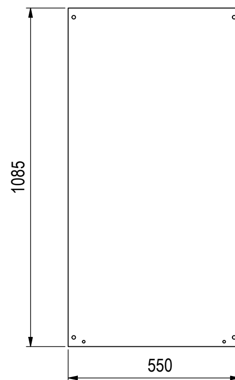
Montageplatte ( 1 : 12 )
