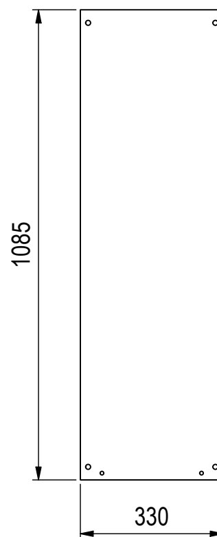
Montageplatte ( 1 : 12 )
