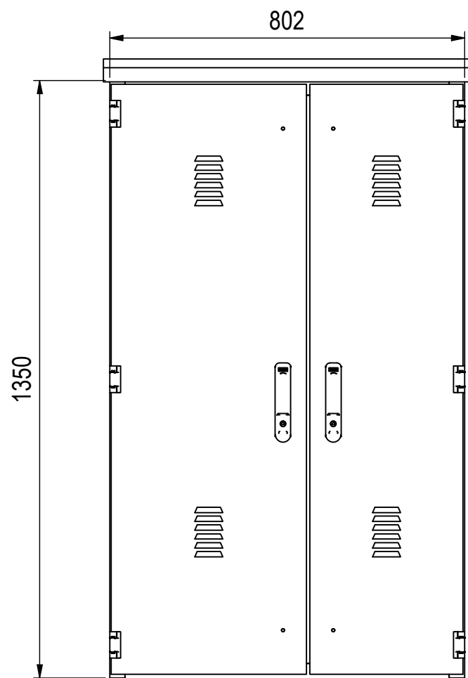
Innenschrank ( 1 : 12 )
