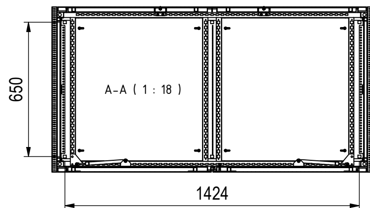
Bodenbefestigung □14mm
