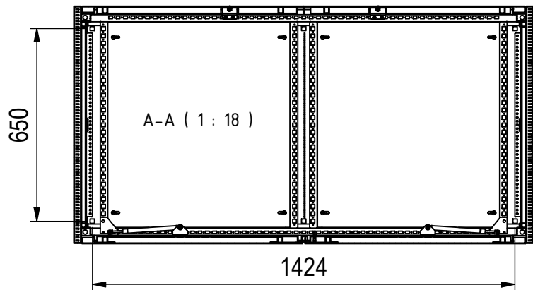
Bodenbefestigung □14mm
