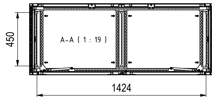
Bodenbefestigung □14mm
