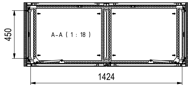
Bodenbefestigung □14mm
