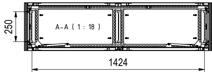
Bodenbefestigung □14mm
