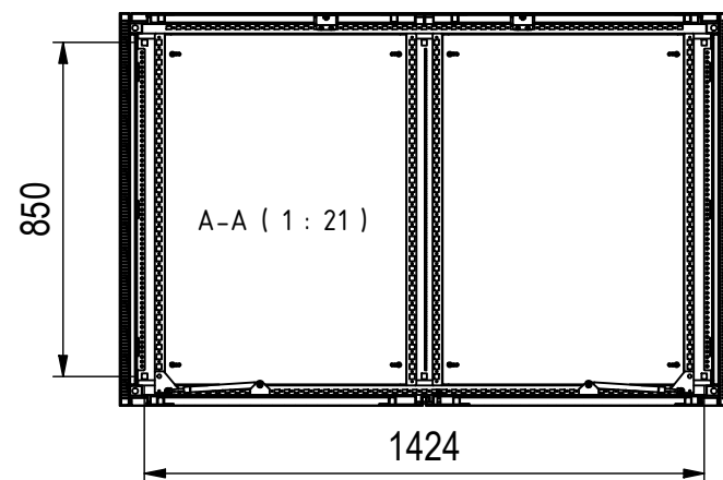
Bodenbefestigung □14mm
