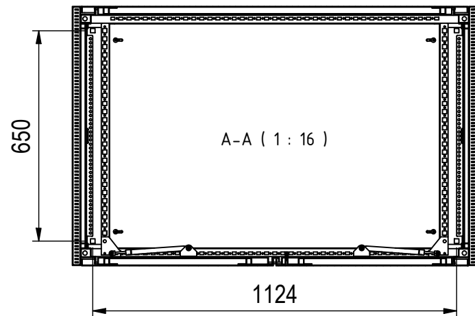
Bodenbefestigung □14mm
