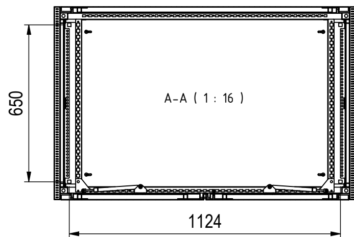
Bodenbefestigung □14mm
