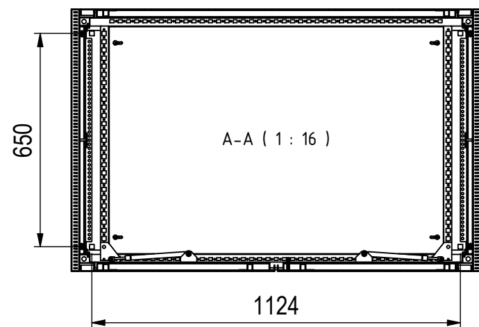
Bodenbefestigung □14mm
