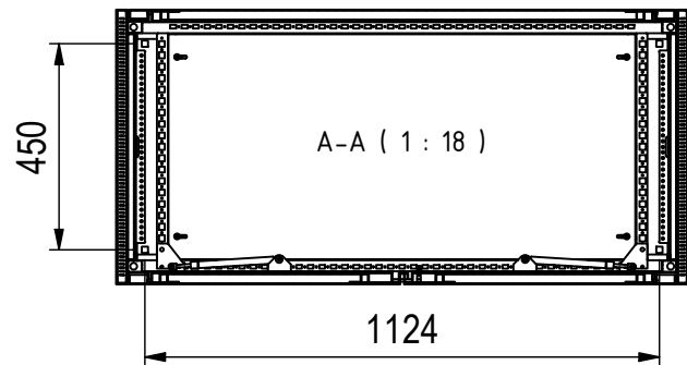
Bodenbefestigung □14mm
