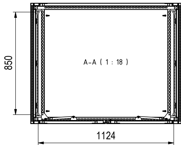
Bodenbefestigung □14mm
