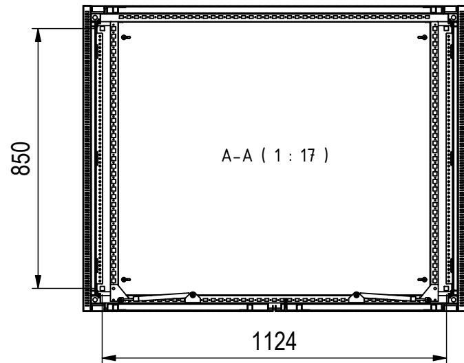
Bodenbefestigung □14mm
