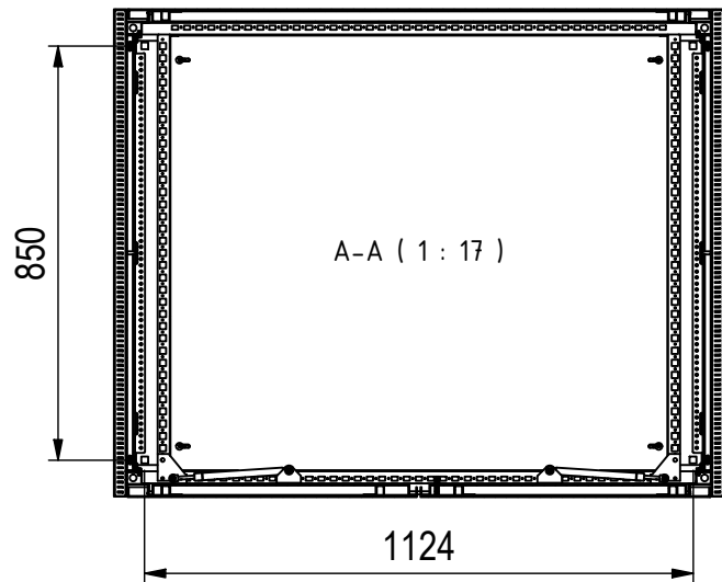
Bodenbefestigung □14mm
