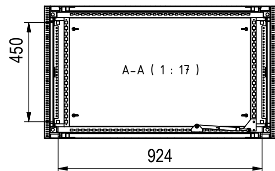
Bodenbefestigung □14mm
