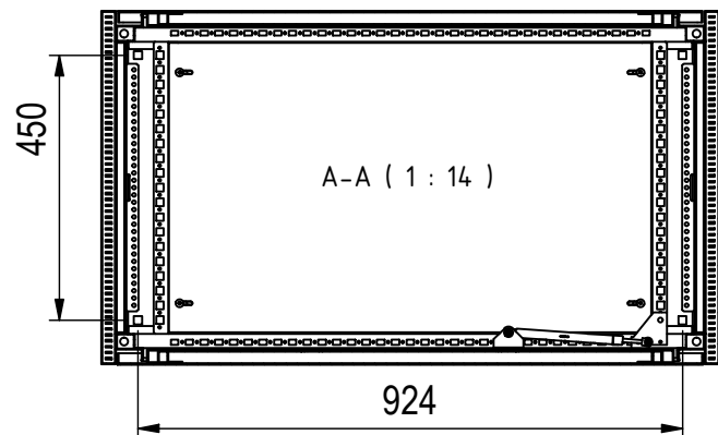
Bodenbefestigung □14mm
