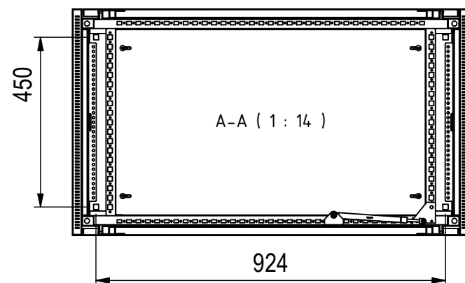
Bodenbefestigung □14mm
