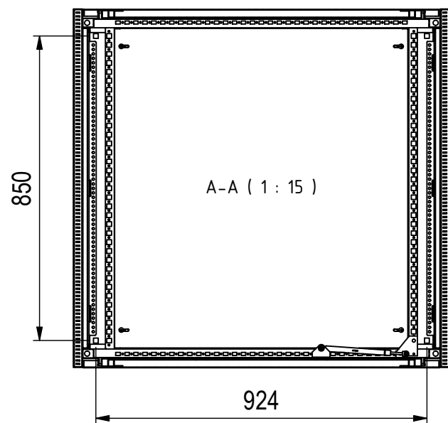
Bodenbefestigung □14mm
