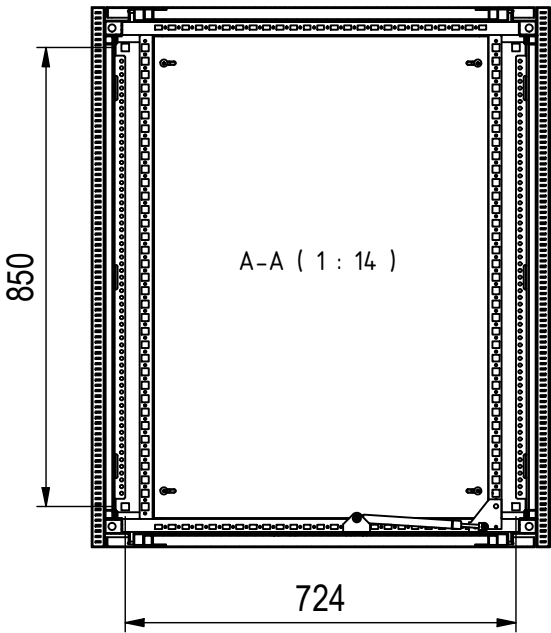
Bodenbefestigung □14mm
