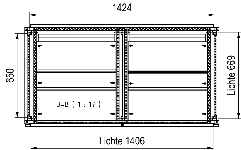
Bodenbefestigung □14mm
