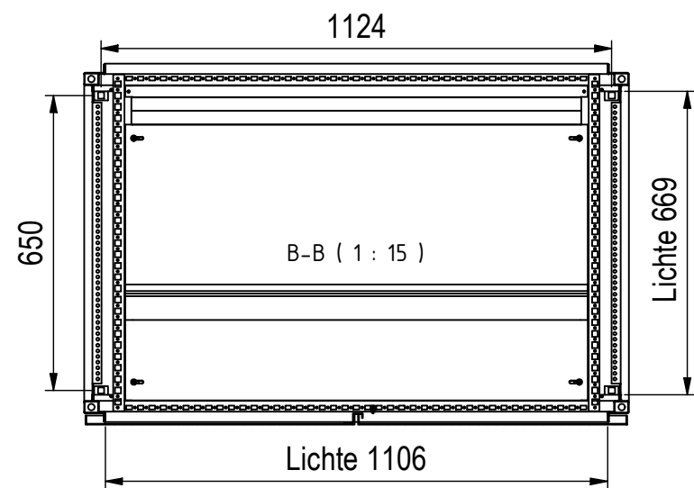
Bodenbefestigung □14mm
