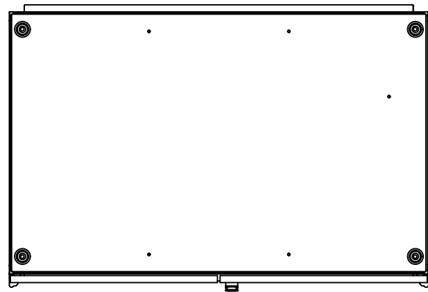
Bodenbefestigung □14mm
