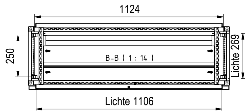
Bodenbefestigung □14mm
