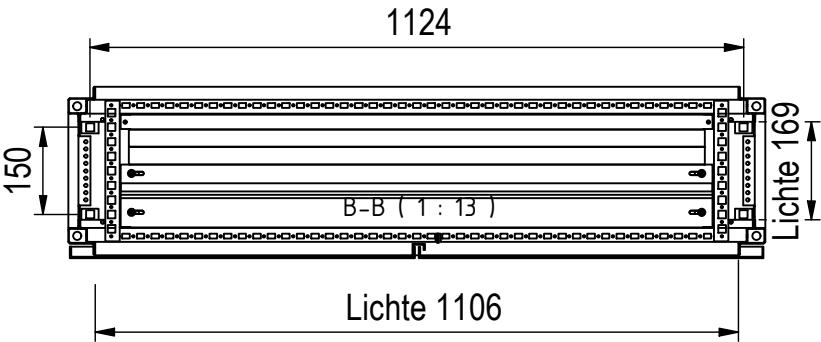
Bodenbefestigung □14mm
