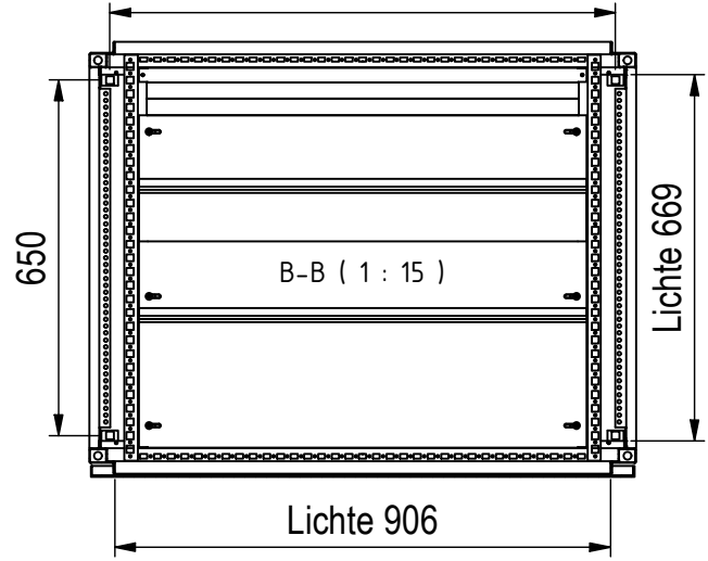
Bodenbefestigung □14mm 924
