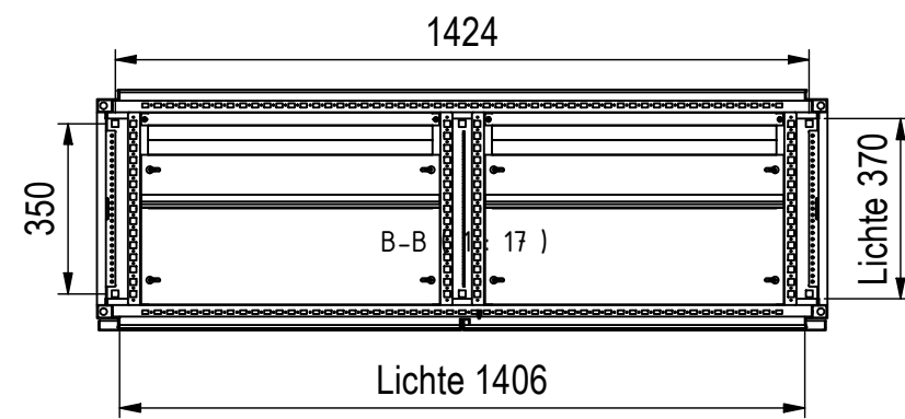
Bodenbefestigung □14mm
