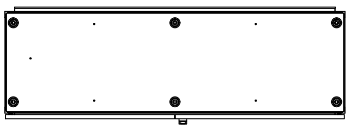
Bodenbefestigung □14mm
